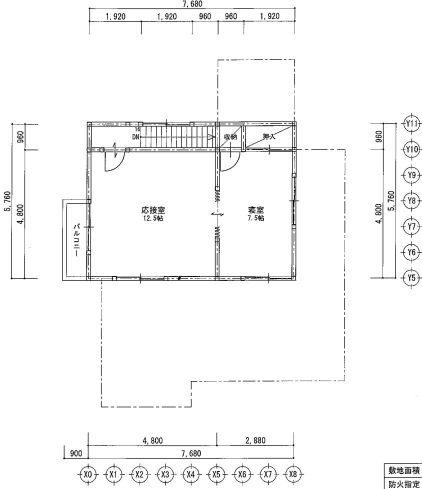
2階平面図
